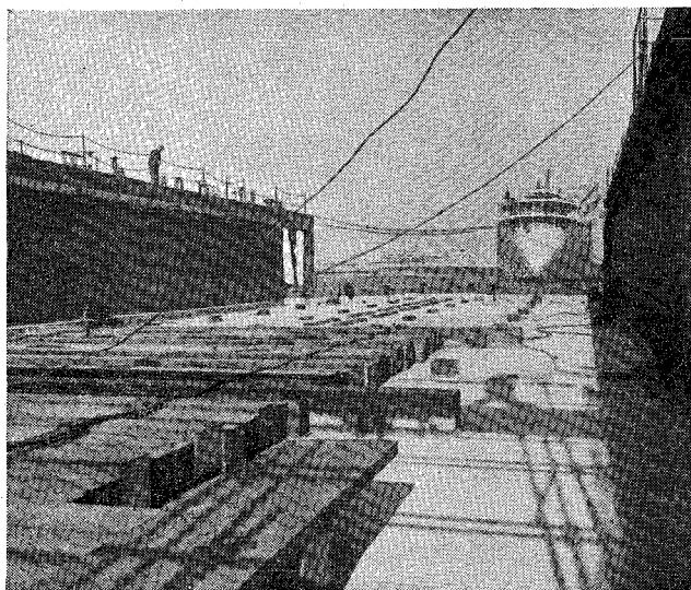
Drijvend dok van beton, waarin de grootste schepen gedokt kunnen worden.
