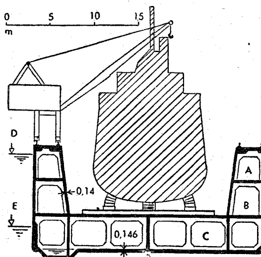
Doorsnede van betonnen dok, met er in opgenomen: schip en loopkraan.
