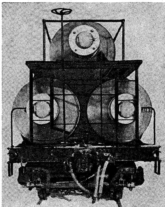
Speciaal voor het transport van helium, gebouwde tankwagen. In gebruik in Amerika.
