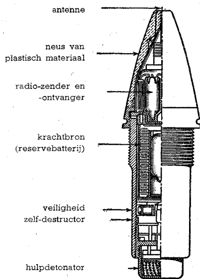
Doorsnede V.T. fuse (naar „Discovery“)
