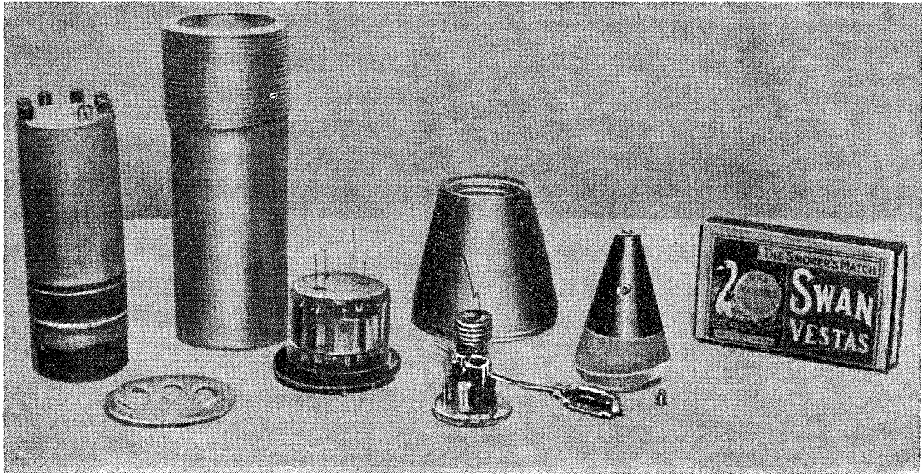
Onderdelen der V.T. fuse. Afmetingen te vergelijken met die van het lucifersdoosje.
