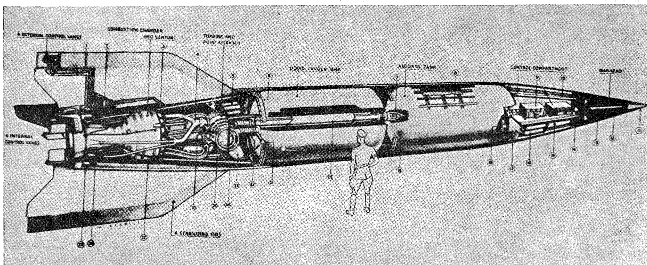
Doorsnede van V 2: V.l.n.r. (bovenkant): vier uitwendige en vier inwendige vinnen voor het houden van de richting; tusschen 2 en 3: verbrandingskamer; tusschen 4 en 5: turbine en pompen; tusschen 6 en 7: tank voor vloeibare zuurstof; 8: tank voor alcohol; 9 en 10: controle-apparaten; aan de punt: bomlading. Onderkant (achter): vier vinnen voor het stabiliseeren. (naar „Discovery” Juni 1945)
